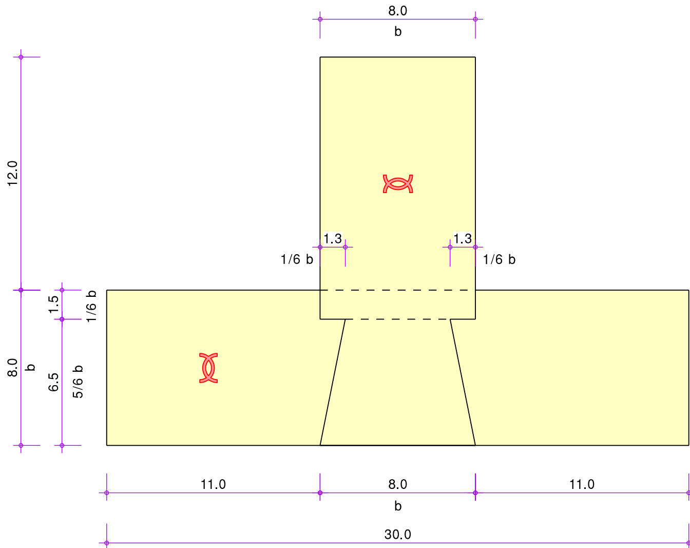
Draufsicht
