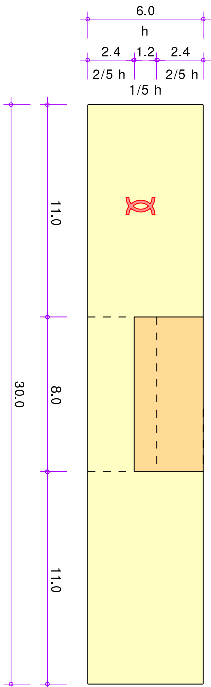
Vorderansicht
