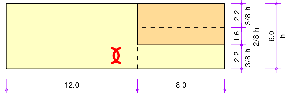
Vorderansicht
